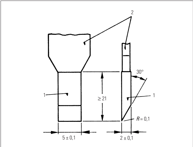
Fig. 1. Electrode a)
