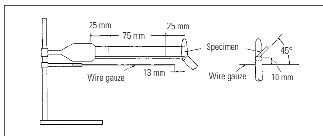
Fig. 1. Test apparatus
